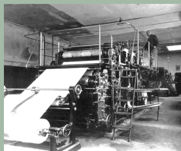
Wielobarwna maszyna rotacyjna z mechanizmem do druku ilustracji. W ciągu godziny drukowała dwustronnie 14000 numerów gazety o objętości 16 stron.
